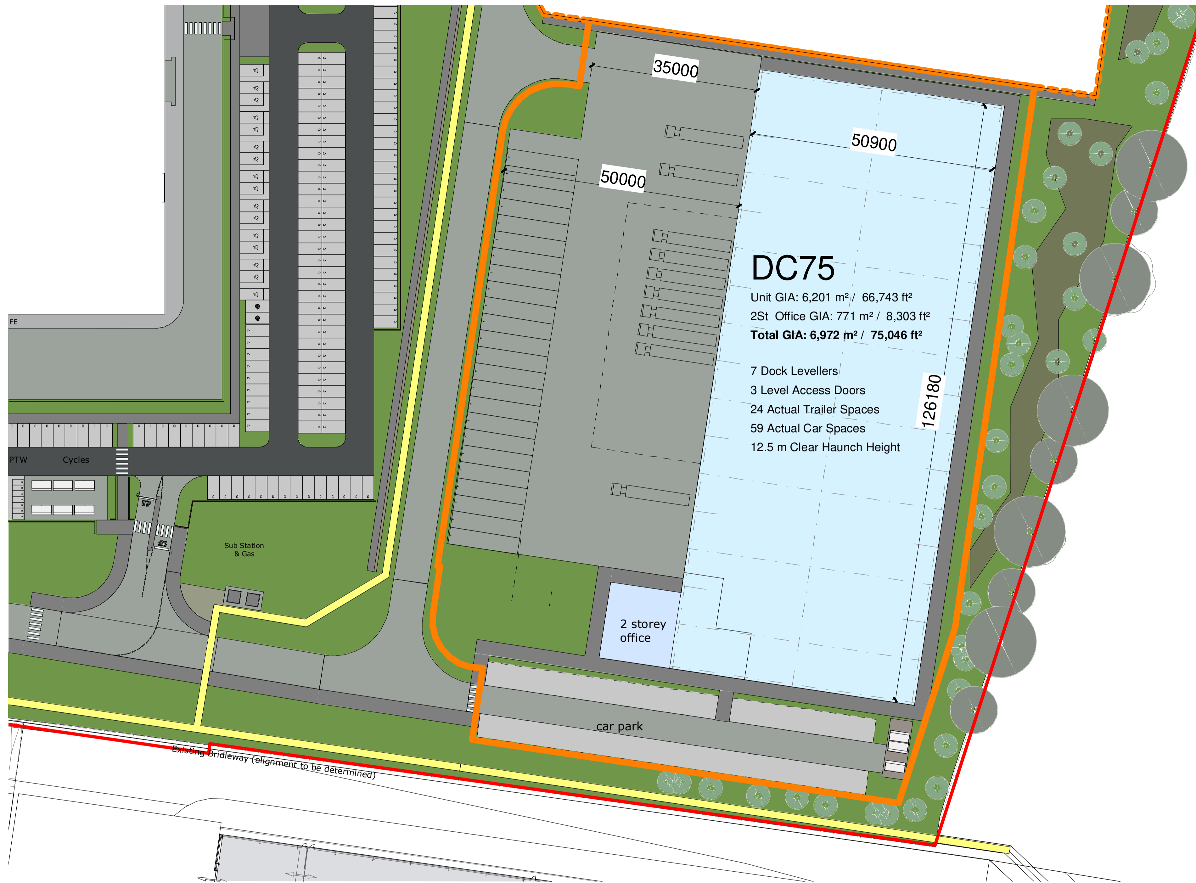
Site Layout 1 : 500
